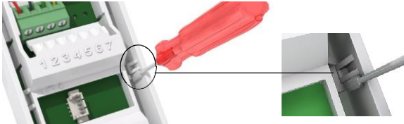
Şekil 4 – Ana Ünitenin çıkarılması
