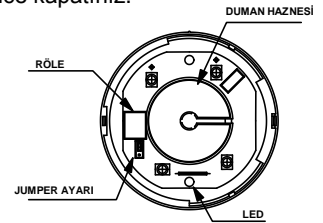
Şek. 3 Ön kapak açırken detektör yapısının şeması.
