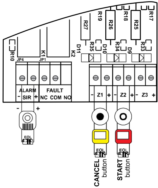
Şekil 7. Zon Çiftleme Fonksiyonu
