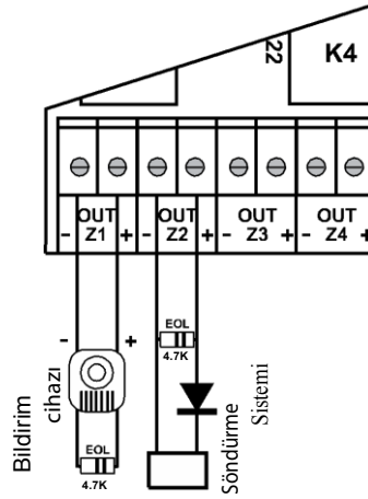
Şekil 8. Zon Çiftleme için Röle bağlantıları (Bölge 1 & 2)
